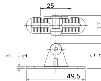
Herraje de puerta de aluminio
