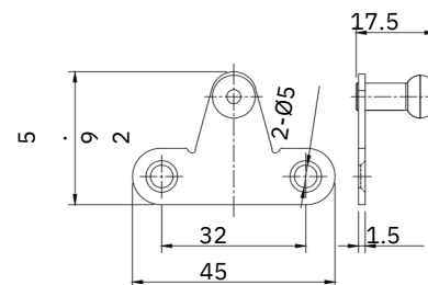
Herraje de puerta de aluminio
