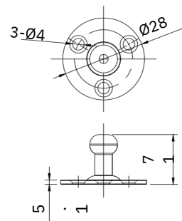
Herrajes para puertas laterales
